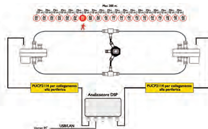
Schema di configurazione sistema PPS™.
