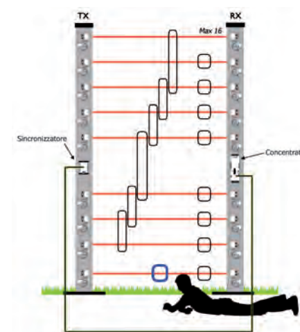
Schema di configurazione sistema IPS™.
