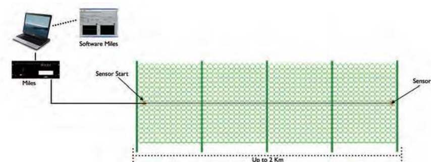
Schema di configurazione sistema MILEST TM | Versione per recinzioni
